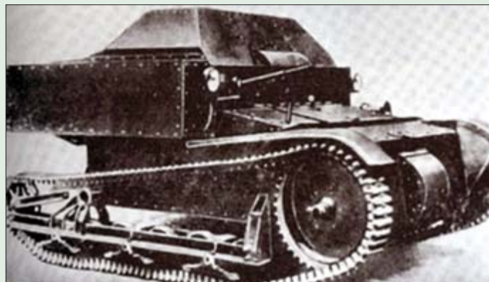
Танкета Т-27а
